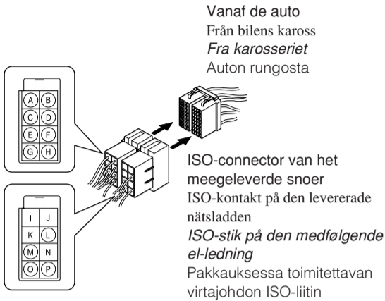
Aanzicht vanaf het snoer Sett från ledarsidan Set fra ledningssiden Näkymä johdon puolelta
